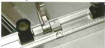
Detailansicht Gehrungsanschlag
