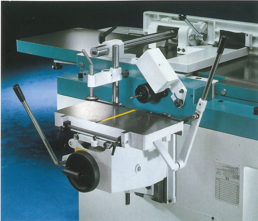
Gruppo cavatrice (a richiesta) Mortising attachment (on request) Groupe mortaiseuse (auf anfrage) Langlochbohrereinrichtung (sur demande) Dispositivo de taladrar (a pedido)
