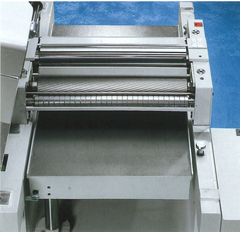
Guida supplementare mobile per lavorazione pezzi piccoli. Additional moving fence to work short pieces. Guide supplémentaire mobile pour usinage des pièces petites. Schwenkbarer Hilfsanschlag für Bearbeitung der kleinen Werkstücke. Guia extra mobile para el trabajo de piezas pequeñas.
