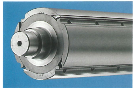
Option • Albero a pialla "MONOBLOC" con coltelli Torsa • Planer shaft "MONOBLOC" with Torsa Knives • Arbre "MONOBLOC" avec couteaux Torsa "MONOBLOC" • Messerhobelwelle mit Torsa-Messern • Eje "MONOBLOC" con cuchillas Torsa
