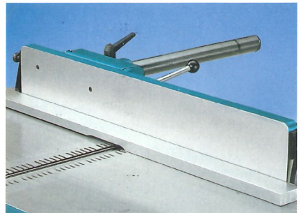
Guida supplementare mobile per lavorazione pezzi piccoli. Additional moving fence to work short pieces. Guide supplémentaire mobile pour usinage des pièces petites. Schwenkbarer Hilfsanschlag für Bearbeitung der kleinen Werkstücke. Guia extra mobile para el trabajo de piezas pequeñas.
