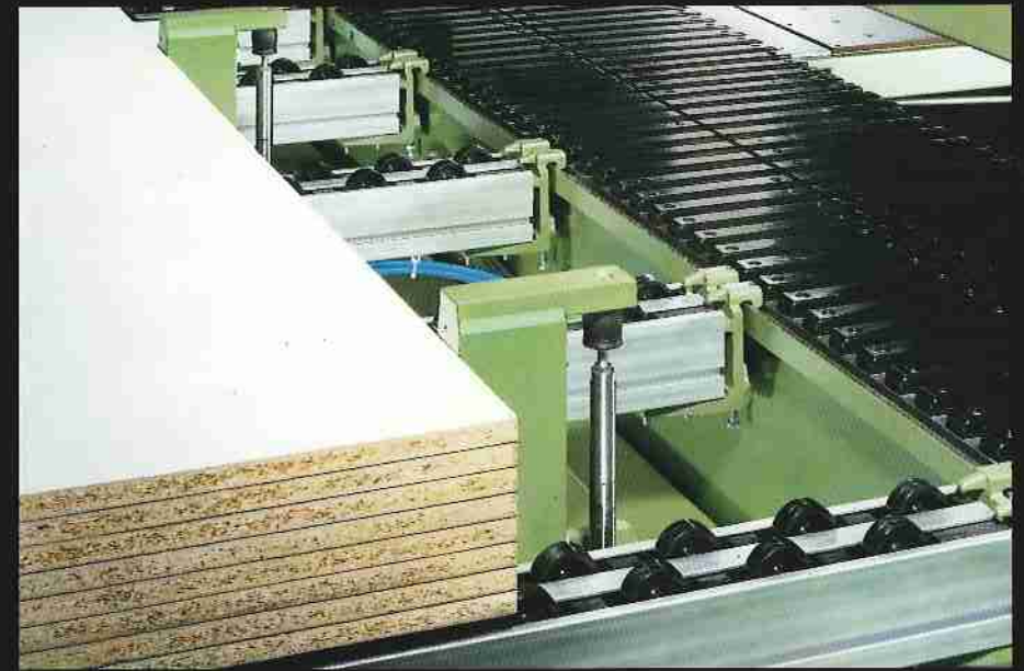
Platten Ausrichtvorrichtung Panel aligning device Dispositif d'alignement de panneaux Dispositivo de alineación de tableros
