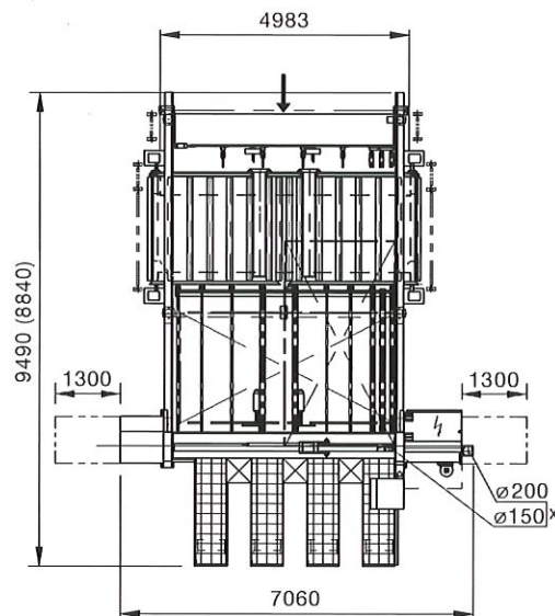
Maße beziehen sich auf die Type HPL 11/43
