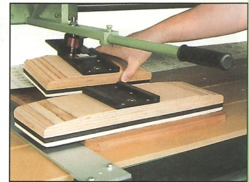
Handgefertigte Schleifschuhe 450 / 650 mm
