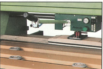
Vakuumsauger für kleine und dünne Werkstücke
