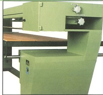
Kröpfung 550 x 310 mm im rechten Maschinenständer
