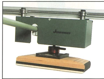
Komfort-Schleifaggregat mit Gleitschielenführung
