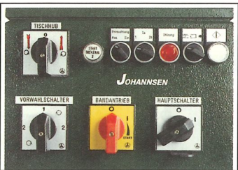
Schaltpult der T 95 AUTOMATIK
