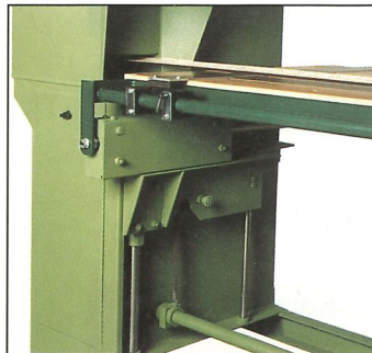
Komfort-Schleifaggregat mit Gleitschielenführung
