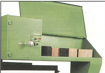
Ablage mit Klappe für Schleifschuhe und Werkzeug im rechten Maschinenständer
