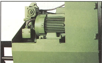
Bandantriebsmotor und Getriebemotor für Tischhöhenverstellung
