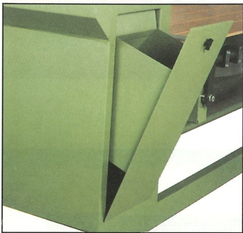
Stauraum für Schleifbänder im linken Maschinenständer
