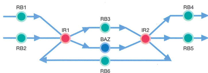
Vermaschte Materialflußstruktur (Beispiel-Layout)
