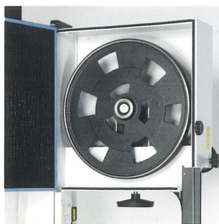
HB 400-700 mit Vollgußrädern und endlosen Schnellwechselbandagen
