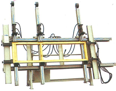
Strettoio tipo DE Frame press type DE Cadreuse type DE Banco de armar tipo DE Rahmenpresse Typ DE
