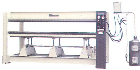
Pressa a caldo C/6 (disponibile anche con piani a freddo S/6) C/6 hot press (cold version too S/6) Presse a chaud C/6 (disponibile aussi a froid S/6) Prensa platos calientes C/6 (disponibile con platos frios S/6) Heizplattenpresse C/6 (auch in kalter Ausführung S/6)
