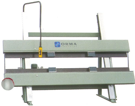
Scambio a barra unica tipo EUROPA Frame press type EUROPA with one horizontal pressing beam Cadreuse a poutre type EUROPA Banco de armar con traviesa unica tipo EUROPA Rahmenpresse mit einem waagrechten Träger Typ EUROPA
