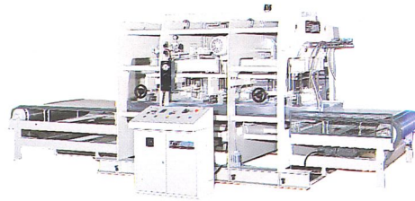
Presse per la lavorazione del poliuretano tipo PXE Presses for poliurethane type PXE Presses pour poliurethane type PXE Prensa para el polyuretano tipo PXE Presse Typ PXE zur Bearbeitung von Polyurethan
