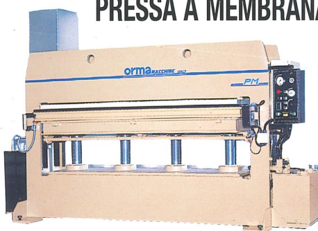
Pressa a membrana tipo PM Membrane press PM Presse a membrane PM Prensa a membrana tipo PM Membran-Formenpresse Typ PM
