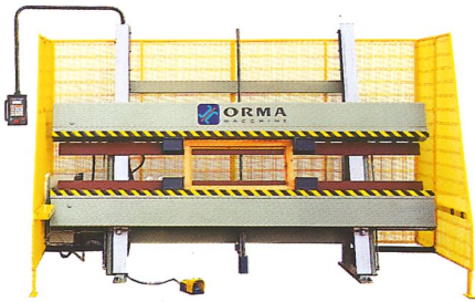
Strettoio EUROPA CNC con centratura elettronica Frame press EUROPA CNC with electronic positioning Cadreuse EUROPA CNC avec centrage électronique Banco de amar EUROPA CNC con centrado electrónico Rahmenpresse EUROPA CNC mit automatischer Zentrierung
