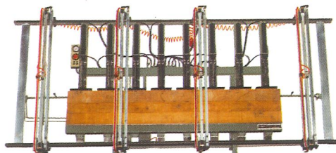
Strettoio per la produzione di travi lamellari Frame press for lammellar beam production Cadreuse pour la production de poutres lamellaires Rahmenpresse für massivholzverleimung und lamellierung Banco para la producion de vigas laminares
