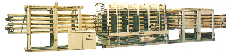
Linea di pressatura in ciclo continuo Multidaylight through feed press (end loading) Ligne a plaquer en continu Linea de prensado en ciclo continuo Durchlaufpreßanlage
