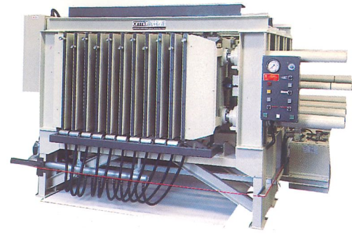
Presse per la lavorazione del poliuretano tipo PXE Presses for poliurethane type PXE Presses pour poliurethane type PXE Prensa para el polyuretano tipo PXE Presse Typ PXE zur Bearbeitung von Polyurethan
