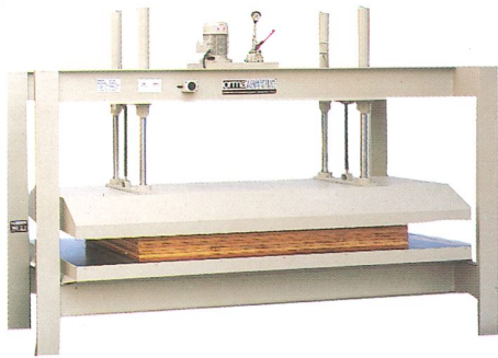
Pressa a freddo P 25/4 (disponibile anche con piani a caldo PCL 25/4) P 25/4 cold press (hot version too PCL 25/4) Presse a froid P 25/4 (disponibile aussi a chaud PCL 25/4) Prensa en frio P 25/4 (disponibile con platos calientes PCL 25/4) Kaltpresse P 25/4 (auch mit Heizplatten, Ausführung PCL 25/4)
