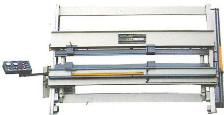
Strettoio SU/FUTURA a ricerca automatica Frame press SU/FUTURA with automatic positioning Cadreuse SU/FUTURA a recherche automatique Banco de amar con busqueda automatica de la madera SU/FUTURA Rahmenpresse SU/FUTURA mit automatischer Positionierung
