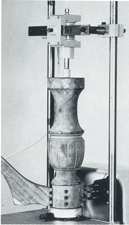
Gruppo divisore e rispettiva applicazione. Special turnable device and specific work application. Dispositif special de blocage et rotation pièce avec son application. Sonderdrehvorrichtung und ihren Arbeitseinsatz.
