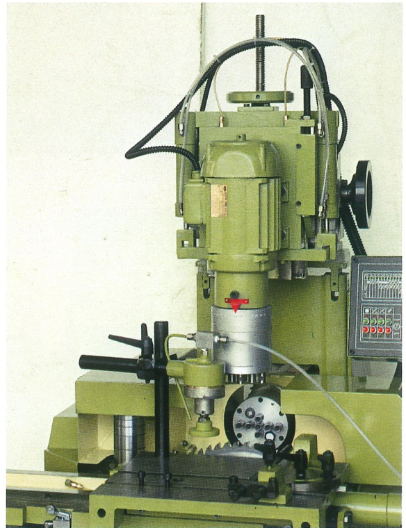
Unità di foratura verticale applicabile sulla PADE 1000/N. Vertical boring unit that can be fitted on machine PADE 1000/N. Unité de perçage verticale applicable sur la machine PADE 1000/N. Vertikaler Bohraggregat einsetzbar an Maschine PADE 1000/N.
