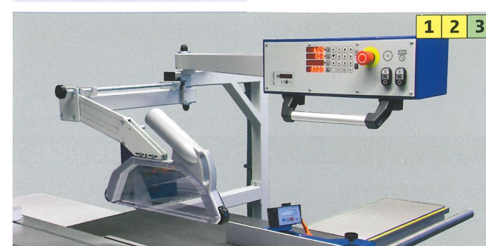
Schaltung oben mit wegschwenkbarer Schutzhaube zum Schneiden von Korpusteilen
