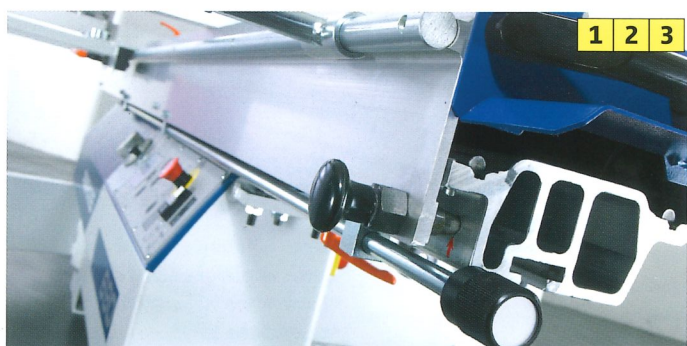
Fernarretierung für Rollwagen
