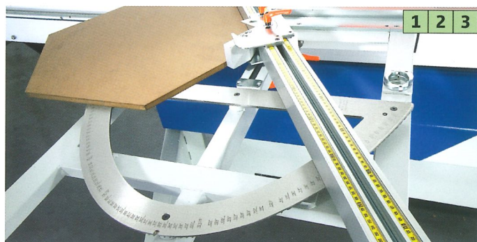
Gehrungs- und Längenanschlag SUPER-GEHRFIX I mit autom. Längenausgleich
