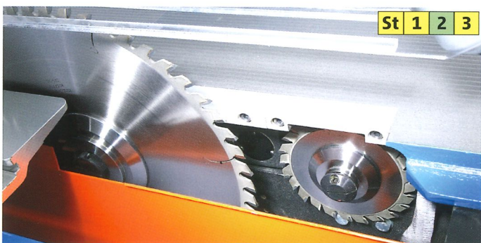
Vorritzaggregat mit elektronischem Parksystem AUTO-EPS kein Verschmutzen des Vorritzsägeblattes in der Parkposition, problemloser Einbau von Hauptsägeblättern > 350 mm, bei eingebautem Vorritzsägeblatt.
