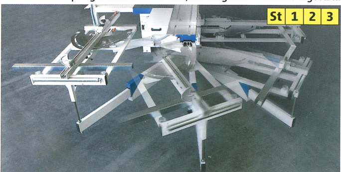
Wegschwenkvorrichtung für Querschlitzen schnelles und ergonomisches Schieben in die Parkposition
