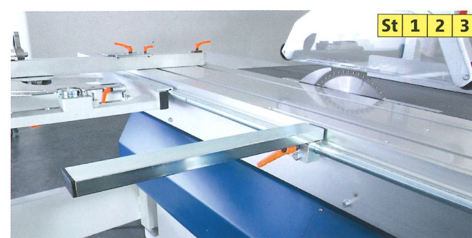
Zusätzliche Auflage für große Platten
