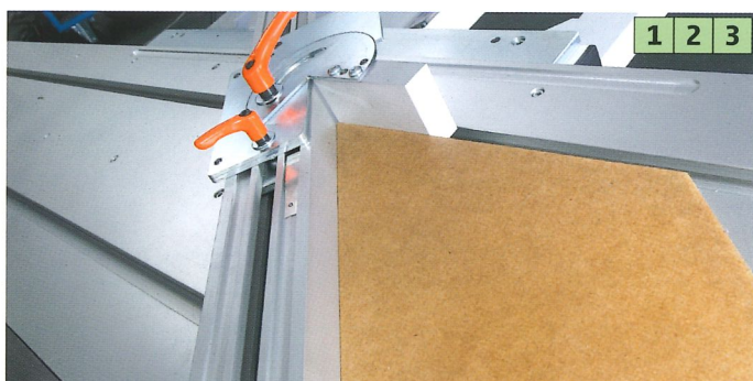
Gehrungs-Hilfsanschlag die Problemlösung beim Anlegen von spitzen und stumpfen Gehrungen
