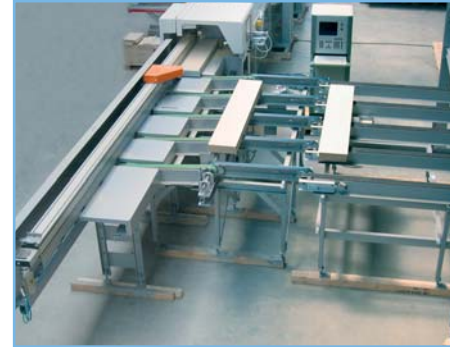
Abb. 36 Variables Ablängen mit CNC-gesteuerter Kappanlage
