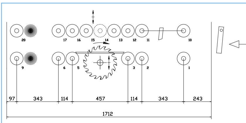
Abb. 22 Schema K34G mit spezieller Rückschlagsicherung
