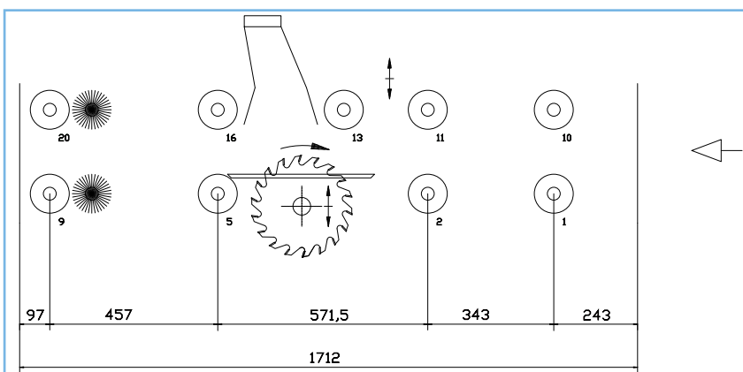
Abb. 23 Schema K34GX ohne Rückschlagsicherung
