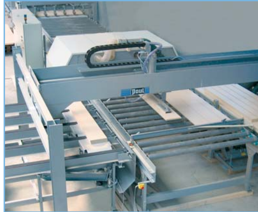
Abb. 35 Stapelbildung der Streifen mit Vakuum-Portal nach Mehrblattsäge K34G/2200 mit automatischer Beschickung
