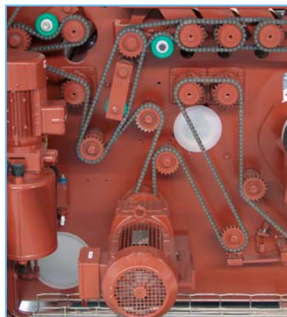
Abb. 19 Vorschubantrieb über Ketten
