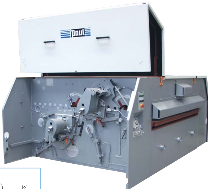
Abb. 29 Modell K34G-OU
