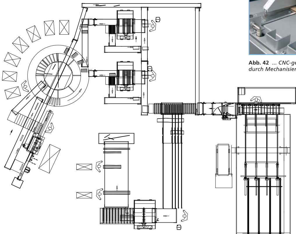
Abb. 43 Zuschnittanlage für Massivparkett (Frieze und Landhausdiele) mit Vorkappen, Auftrennen, Nachkappen und Sortierkarussell
