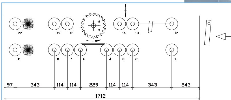
Abb. 26 Schema K34G-O mit spezieller Rückschlagsicherung
