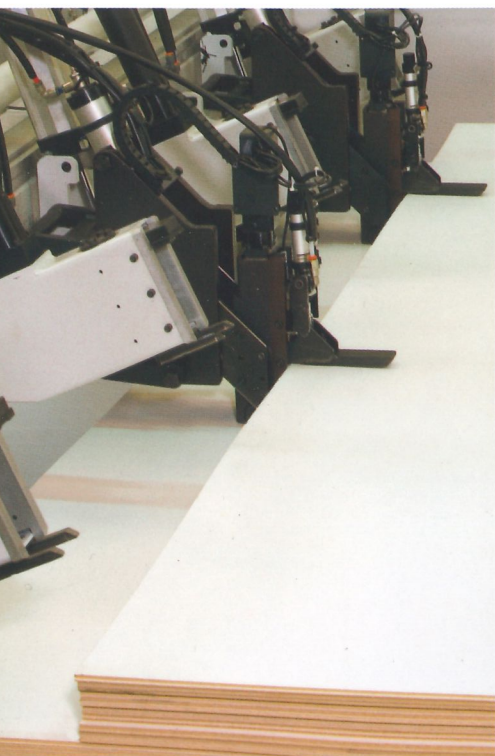
Dispositivo para carga de los paneles delgados Dispositivo para carga dos painéis de fina espessura
