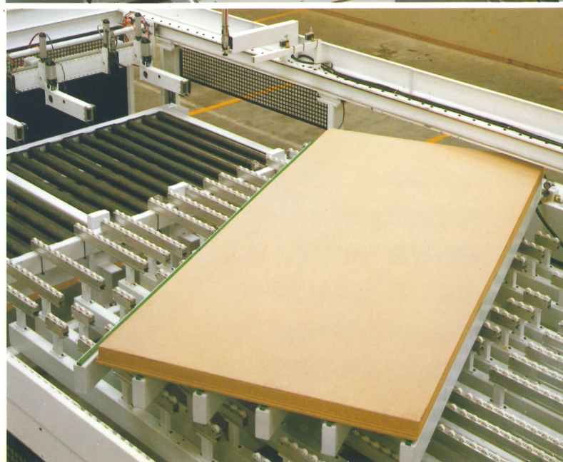
Estación rotante para la ejecución de precorte Estação de rotação para a execução de pré corte
