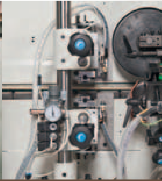
Gluescraping unit
