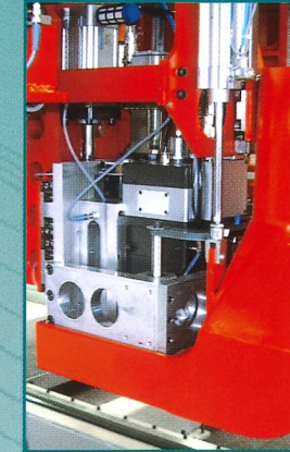
• Hochfrequenz-Spindel mit 50.000/min • high frequency main spindle with 50.000/min
