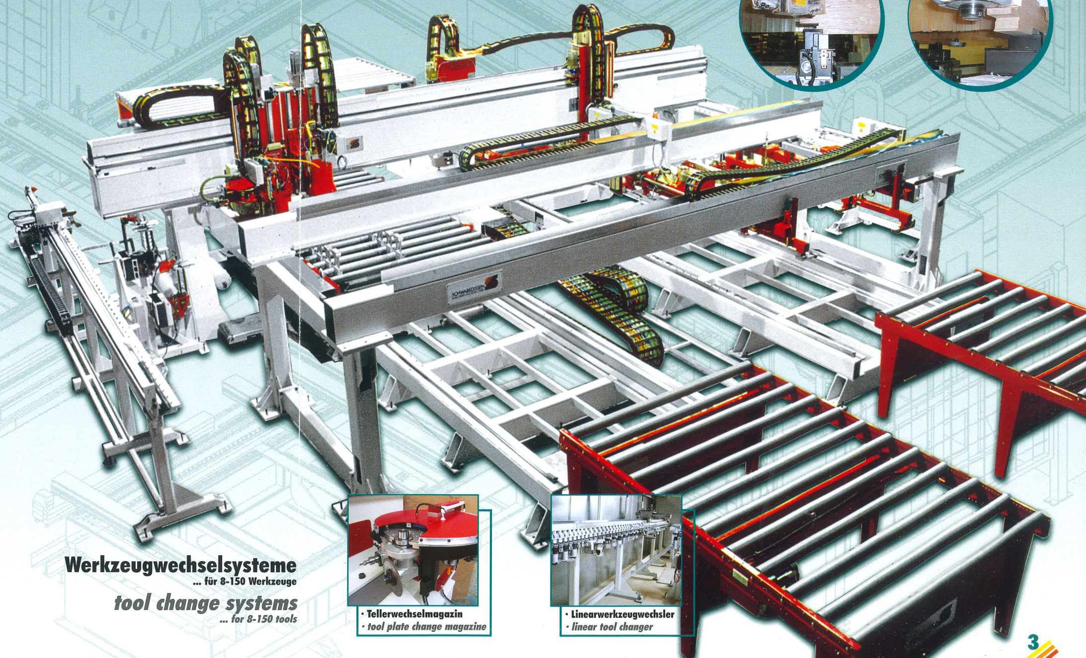
• Langteilmbearbeitung mit selbständigen CNC-Verfahreinrichtungen • long part processing with independant traverse units
