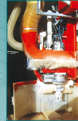
• Standardspindel mit Vectorregelung und Vectorachse • standard main spindle with vector control and vector axis
