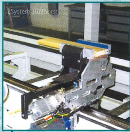
• Langteilmbearbeitung mit selbständigen CNC-Verfahreinrichtungen • long part processing with independant traverse units
