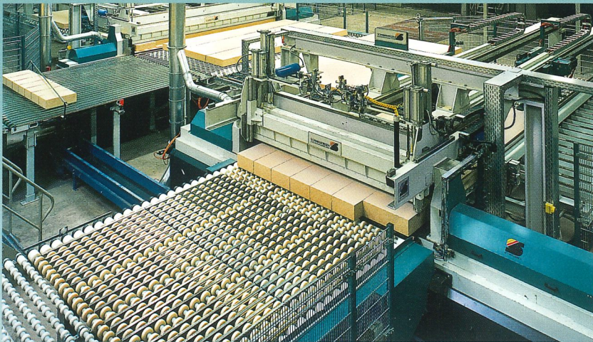
Paketaufteilanlagen in Winkelanordnung angular saw series for books of panels
