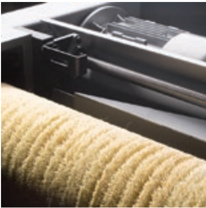
清洁刷由猪鬃及其它不同材料制成,以满足要求最为严苛的板材加工要求。
