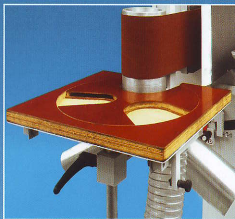
Въртяща се звезда с 2 контактни ролки (KSM 3000) Drehstern mit 2 zusätzlichen Kontaktwalzen (KSM 3000) Device STAR with 2 contact rollers
