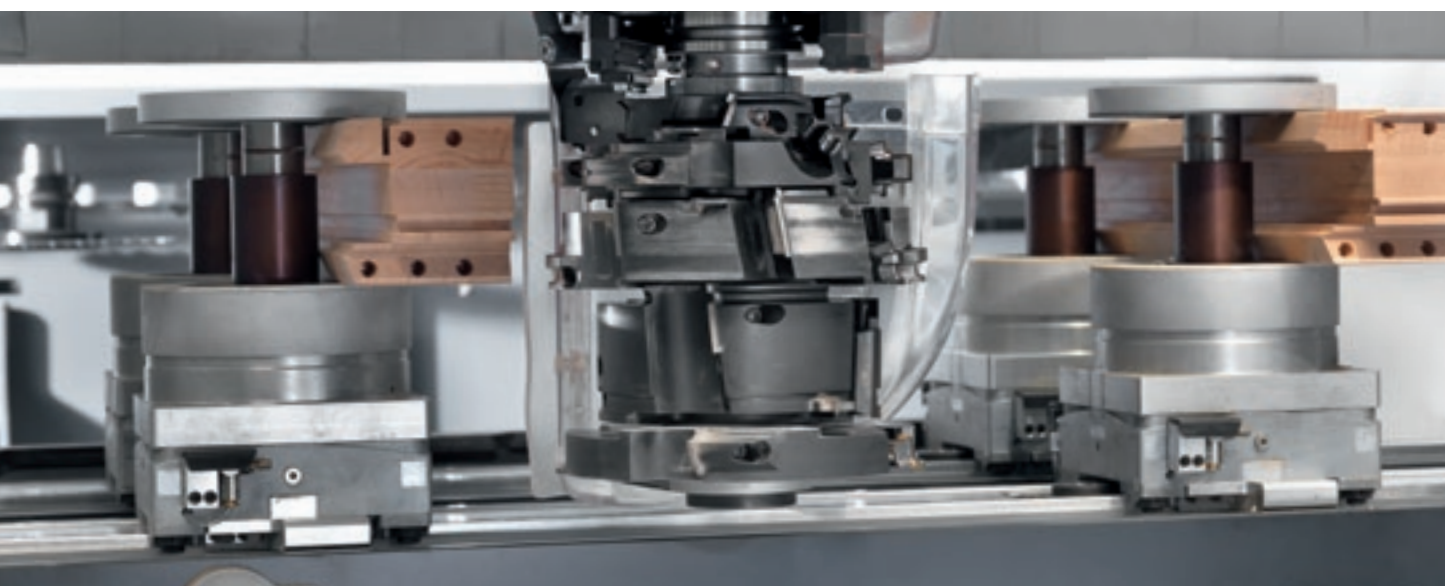
Sistemas de sujeción neumática Uniclamp e Hyperclamp con desenganche rápido para obtener una sujeción rígida y exacta.
