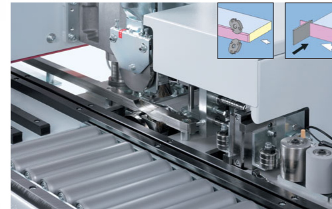
Bündigkappaggregat + Bündigfräsaggregat Agrégat de coupe en bout + agrégat d'affleurage Gruppo intestatore + gruppo refilatore
