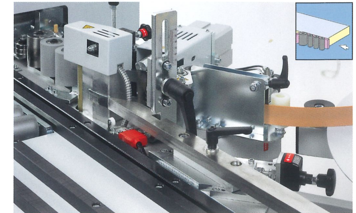
Verleimaggregat + Druckzone Gluing unit and pressure zone Grupo encolador + Zona de presión
