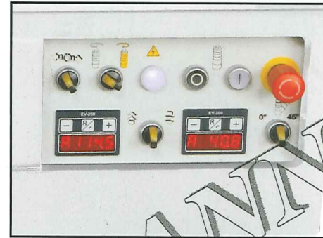
Sollevamento ed inclinazione motorizzati del gruppo toupie con display digitale, in opzione.
