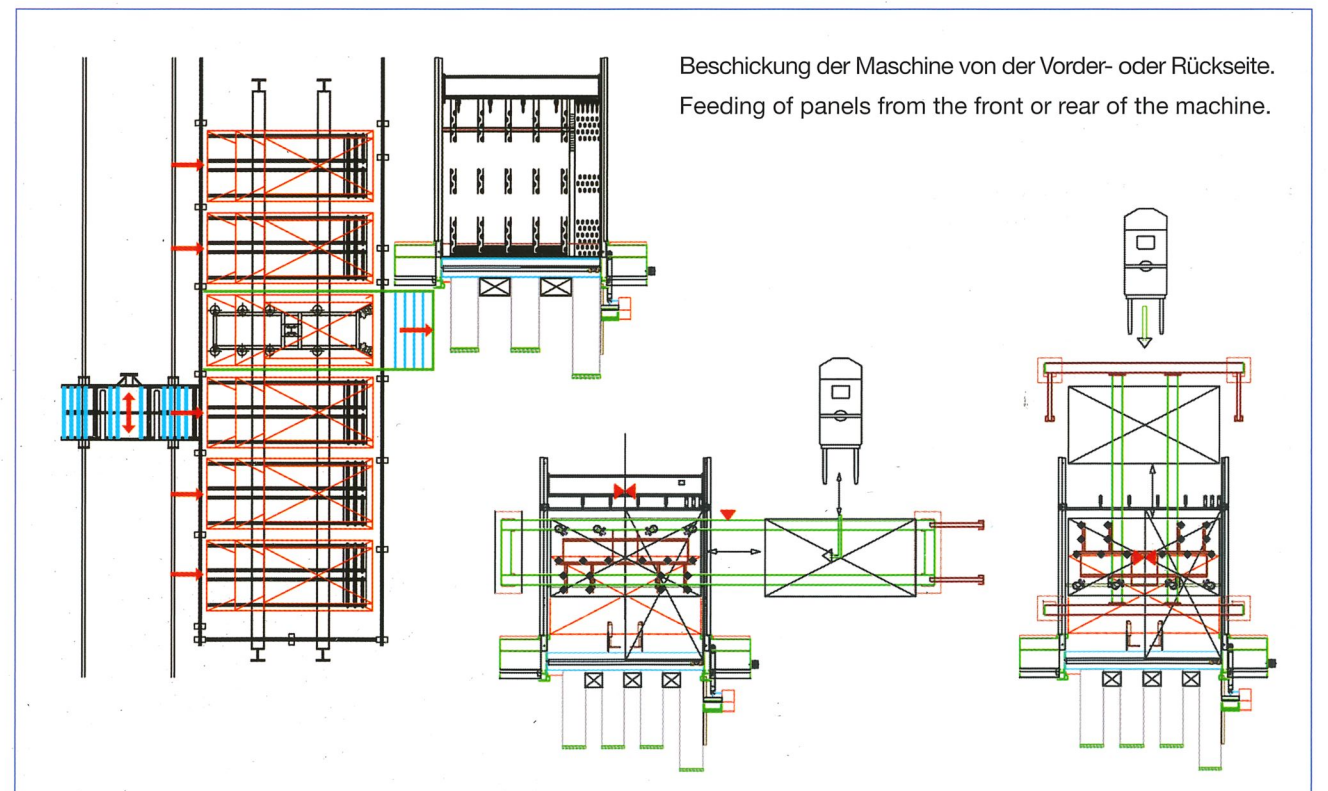
Beispiele individueller Aufstellmöglichkeiten. Examples of individual layouts.
