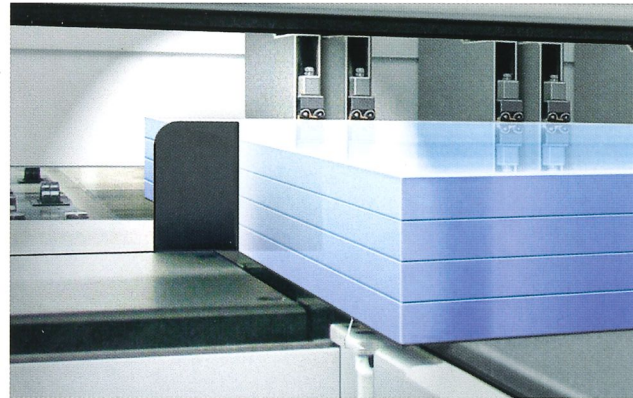
Zentrale Winkelandrückvorrichtung. Einstellbare Kraft und Präzision für jedes Material. Central side pressure device adjustable to any material.
