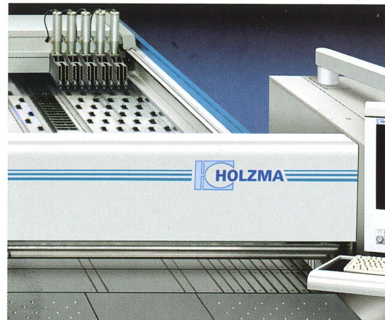
Rollentische: ideal als schonende Materialauflage. Rollertable: ideal for handling sensitive surfaces.
