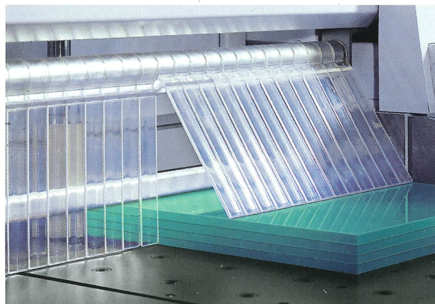
Alles im Blick, alles unter Kontrolle. Transparenter Staub- und Sicherheitsvorhang. Everything visible, everything under control. Transparent dust and safety curtain.
