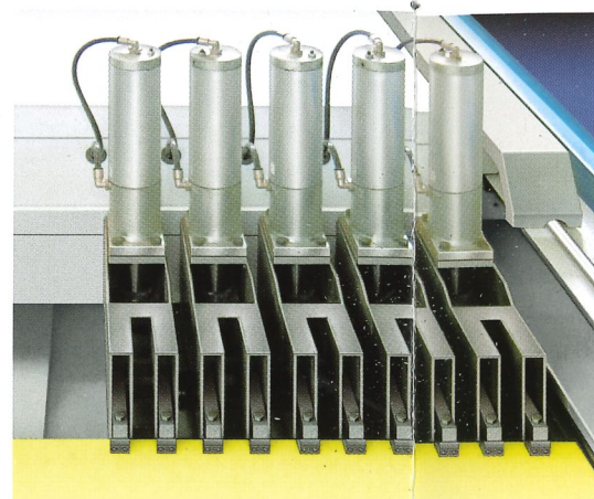
Doppelfinger Spezialspannzangen für glatte Materialien. Double-finger clamps protect sensitive surfaces.
