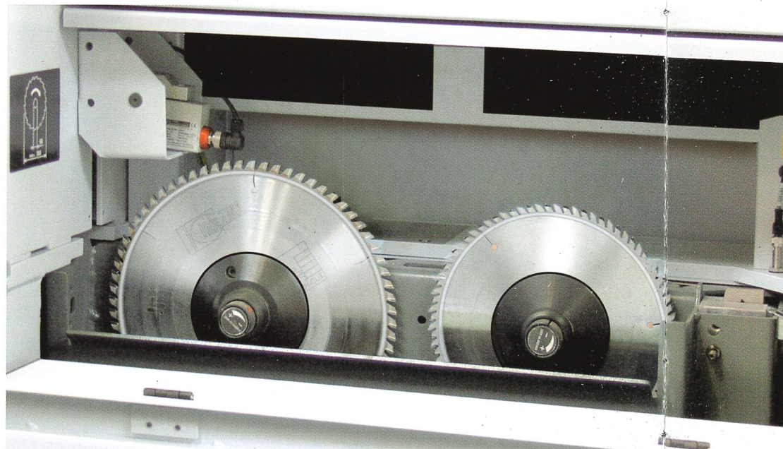
Spezialspannzangen für besonders schmale Tischnuten zum Schneiden dünner Platten. Special clamps with narrow grooves, ensures clean-cutting of thin material.
