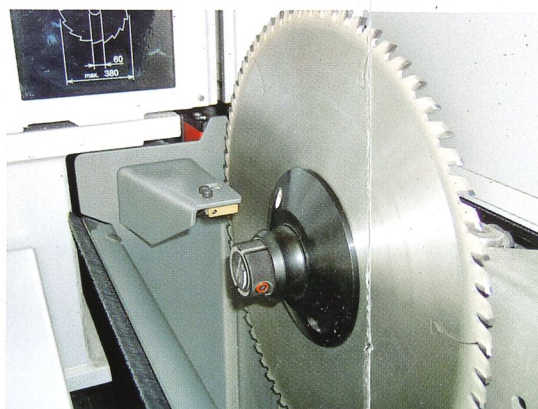
Hauptsägeblatt mit Sprühvorrichtung. Main saw blade with spraying nozzle.
