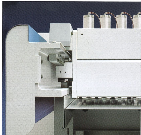
Berührungsloses Mess-System – höchste Positioniergenauigkeit für den Programmschieber. Wartungsfrei, gegen Staub unempfindlich. Magnetic measuring system – unmatched positioning accuracy for the program fence, maintenance free, impervious to dust or wear.
