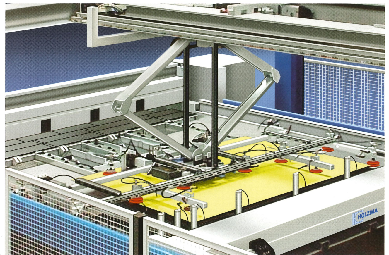
Gesamtsystem Plattenzuschnitt mit automatischer Vakuumbeschickung. Complete "cut-to-size system" with automatic vacuum feeding system.
