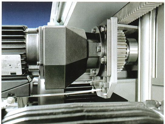
Dynamischer Sägewagenantrieb mit Ritzel und Zahnstange. Dynamic drive of saw carriage by rack and pinion.
