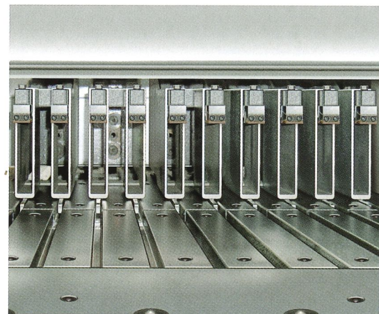
Spezialspannzangen für besonders schmale Tischnuten zum Schneiden dünner Platten. Special clamps with narrow grooves, ensures clean-cutting of thin material.
