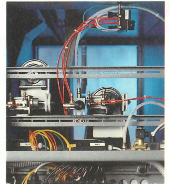
Bandkantensteuerung
