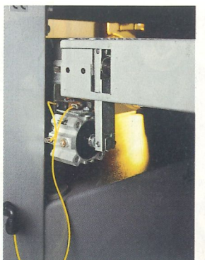
Pneumatische Teppichzentrierung
