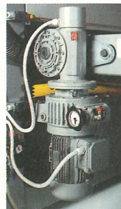
variabler Transport- band-Antrieb
