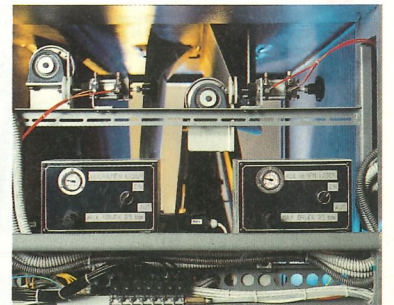
Stufenlose Schleifbandgeschwindigkeit - frequenzgesteuert
