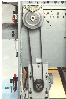
Schleifbandantrieb mit Scheibenbremse
