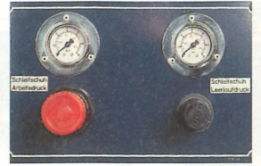
Druckregler AEROSTAT
