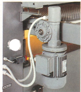
Transportband - Teppichzentrierung - automatisch
