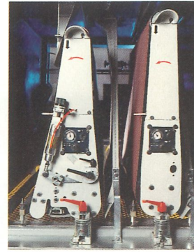
Doppelband 2 RK
