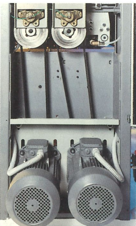
Doppelmotorenantrieb
