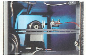
Bandkantensteuerung
