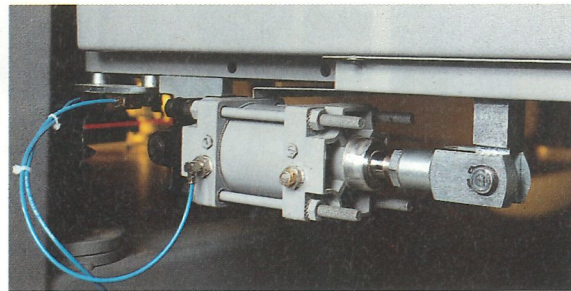
Transportband - Teppichzentrierung - automatisch
