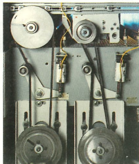
variabler Transport- band-Antrieb
