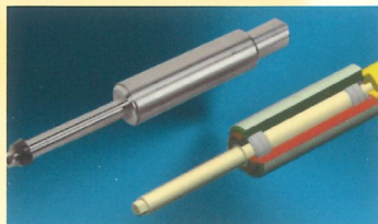
4-fach gelagerte Spindeln für 8000 oder 9000 Upm
