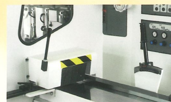
Rückschlagsicherung im Einlauf
