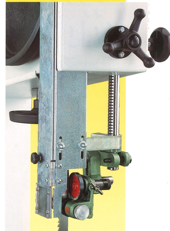
mechanische Höhenverstellung durch Handrad mit Sperritzel
