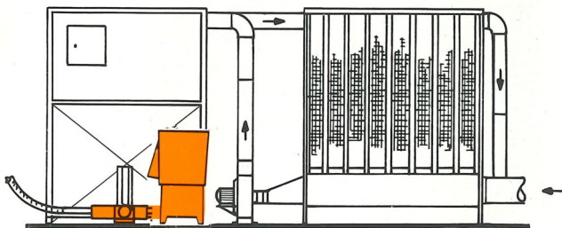
Compacto mit Bunker und Filter für niedrige Raumhöhen
