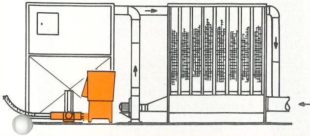
Compacto mit Bunker und Filter für niedrige Raumhöhen
