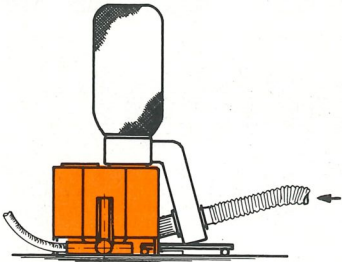
Compacto mit 0,75 m³ Behälter und fahrbarem Absauggerät
