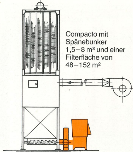
Compacto unter Spänesilo
