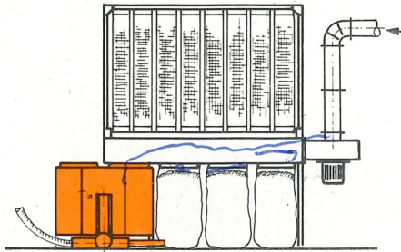
Compacto mit 0,75 m³ Behälter unter Absackanlage
