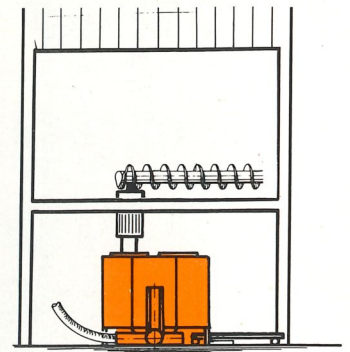
Compacto unter Spänesilo
