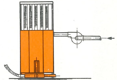
Compacto mit 1,3 m³ Behälter und Filter
