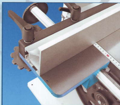
Линеал с финна настройване Feinabstimmung Anschlag Fine adjustable fence
