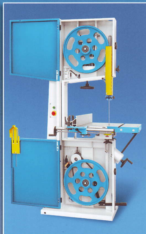
Механично наклоняне на маса Tischschwenkeinrichtung Mechanical tilting of the table
