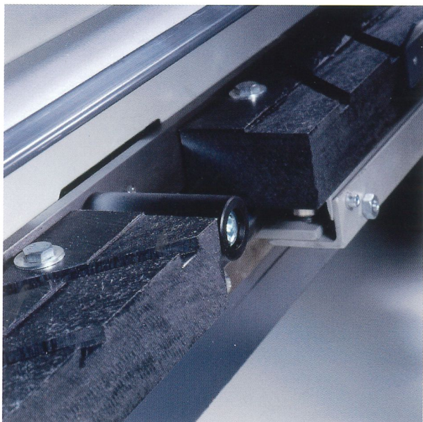
Plan d'appui inférieur sur des blocs en matériaux composites durs, glissants et résistants à l'usure. Galets escamotables pour le chargement et transport des panneaux en option.
