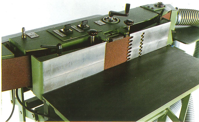
Furnierkantenschleifseite mit Bedienelementen
