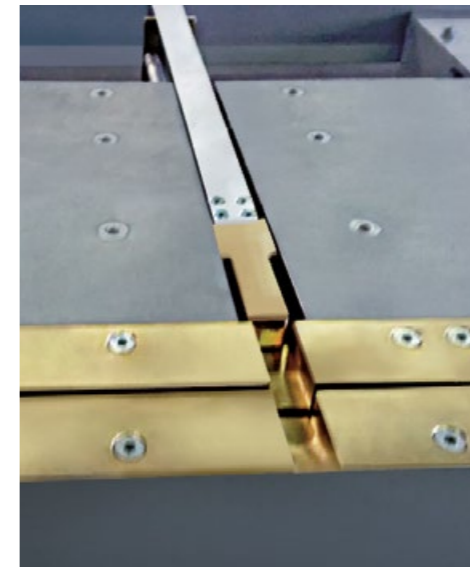
Obturateur de fente de coupe pour les coupes de propreté.
