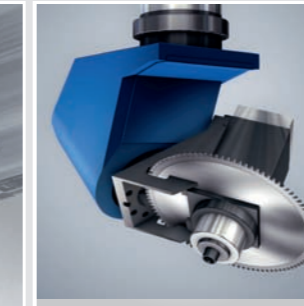
5-Achs-Kopf zum Sägen, Bohren und Profilieren
