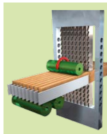
Alimentador de 9 canales
