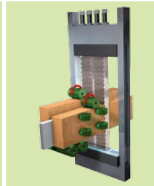
Guía central con rodillos prensos independientes
