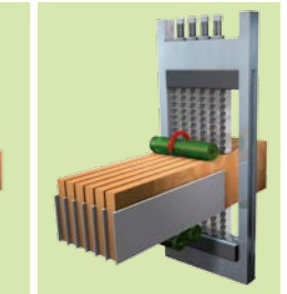
Alimentador de 6 canales
